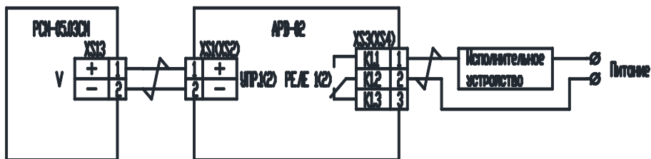
Рис. Г.2 - Подключение APB-02 к расходомеру PCM – 05.03CM с активизированной функцией «Доза»
