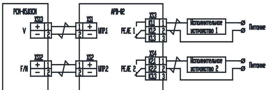
Рис. Г.1 - Подключение APB-02 к расходомеру PCM – 05.03CM с активизированной функцией «Контроль G_{\uparrow} и G_{\downarrow} »
