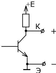
выходной сигнал – «напряжение»
