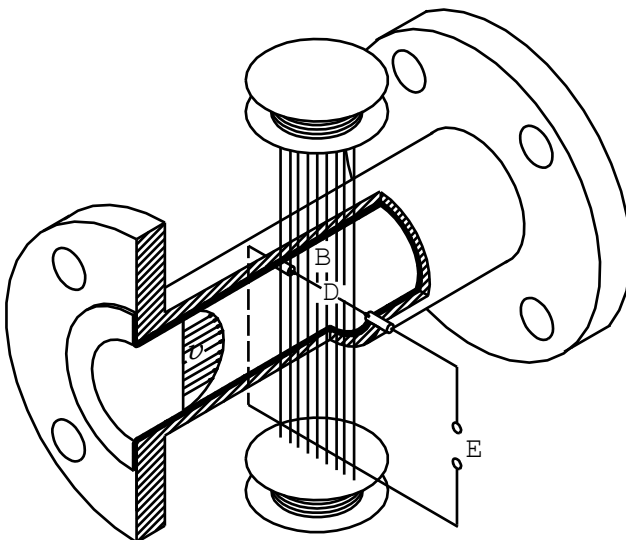
Принцип действия и устройство ППР
